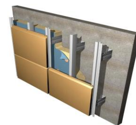
Фасадные кассеты
